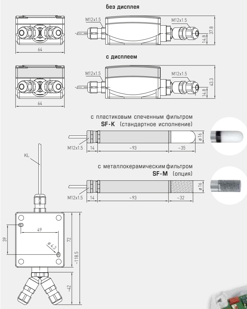
Габаритный чертеж
