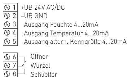
Anschlussbild
