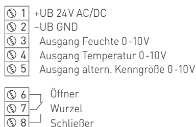
Anschlussbild
