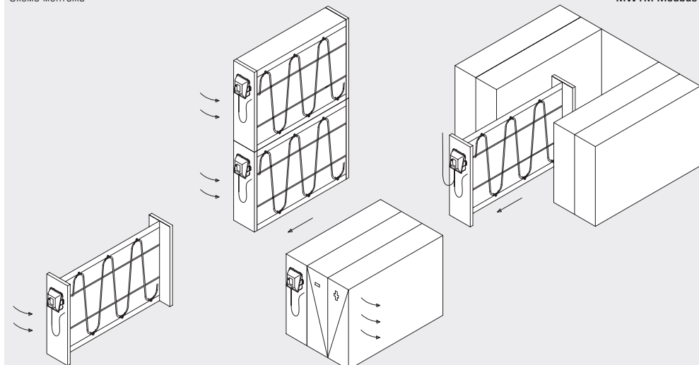
Схема монтажа
