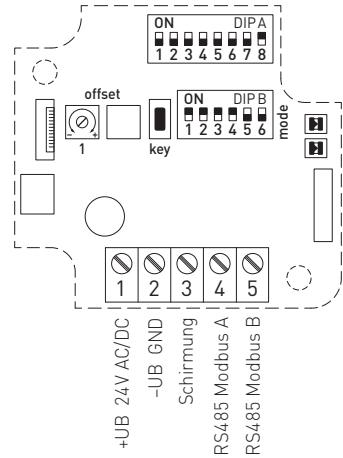
Schaltbild
