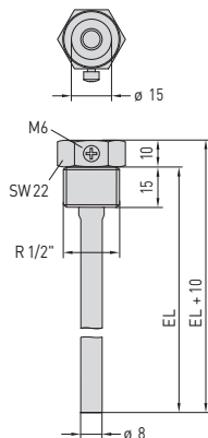
Maßzeichnung TH08-MS/xx Dimensional drawing Plan coté Габаритный чертёж
