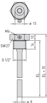
Maßzeichnung TH08-VA/xx Dimensional drawing Plan coté Габаритный чертёж
