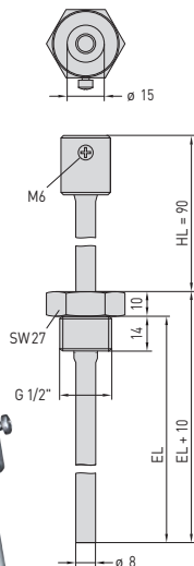
Maßzeichnung TH08-VA/xx/90 Dimensional drawing Plan coté Габаритный чертёж
