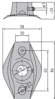
Maßzeichnung MF-15-K Dimensional drawing Plan coté Габаритный чертёж
